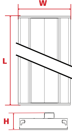
Dimensions : 1' x 4'
